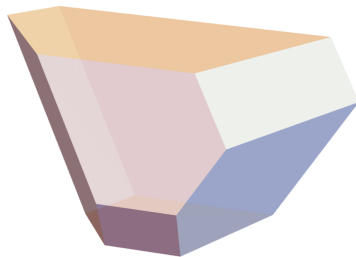
FIGURE 1.1 : La réalisation de Loday de l'associaèdre de dimension trois.
