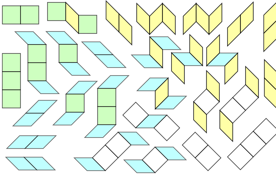
FIGURE 5.2 – Motifs interdits des pavages golden octagonal .
