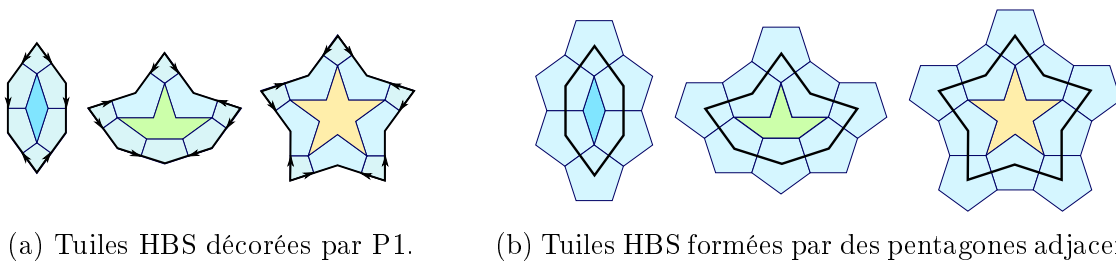
FIGURE 2.7 – Simple correspondance entre tuiles HBS et P1.
